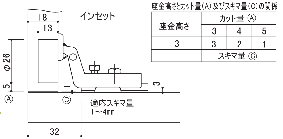
品名: ミニスライド丁番 φ26 インセット システム座 品番: KE011ST030-02 KE011ST030-02-NB パネ無
