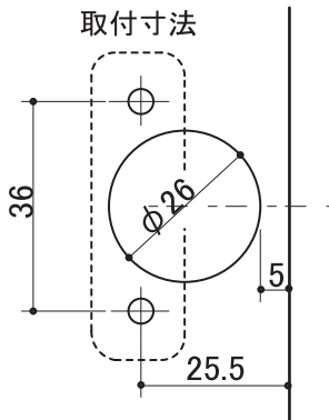
品名: ミニスライド丁番 φ26 インセット システム座 品番: KE011ST030-02 KE011ST030-02-NB パネ無
