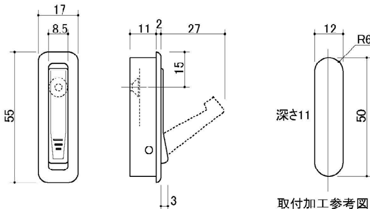
寸法図
