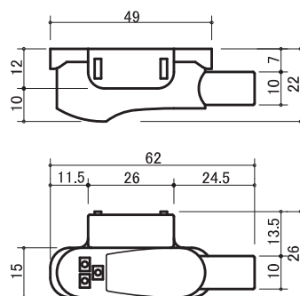
寸法図
